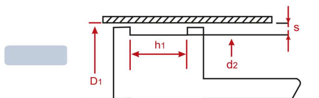
BWR01-P: d2 \times D1 \times h1 \text{ ó } s \times h1
