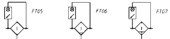
FT05 = filtro con descarga directa G1/8 e indicador visual de bloqueo FT06 = filtro con descarga semiautomática-manual e indicador visual de bloqueo FT07 = filtro con descarga automática/despresurizada e indicador visual de bloqueo
