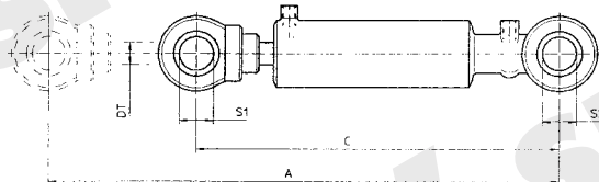
MARTINETTO CON ATTACCHI EQUIDISTANTI
