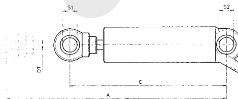
MARTINETTO CON ATTACCHI POSTERIORI
