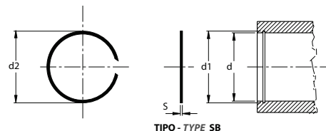
TIPO - TYPE SB
