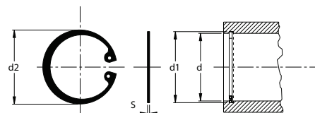
TIPO - TYPE DIN 472 UNI 3654-7437
