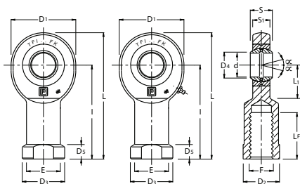
TFI 6 FK - TFI 20 FK TFI 25 FK - TFI 80 FK
