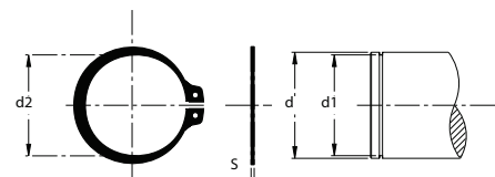
TIPO - TYPE A DIN 471 UNI 3653 - 7435
